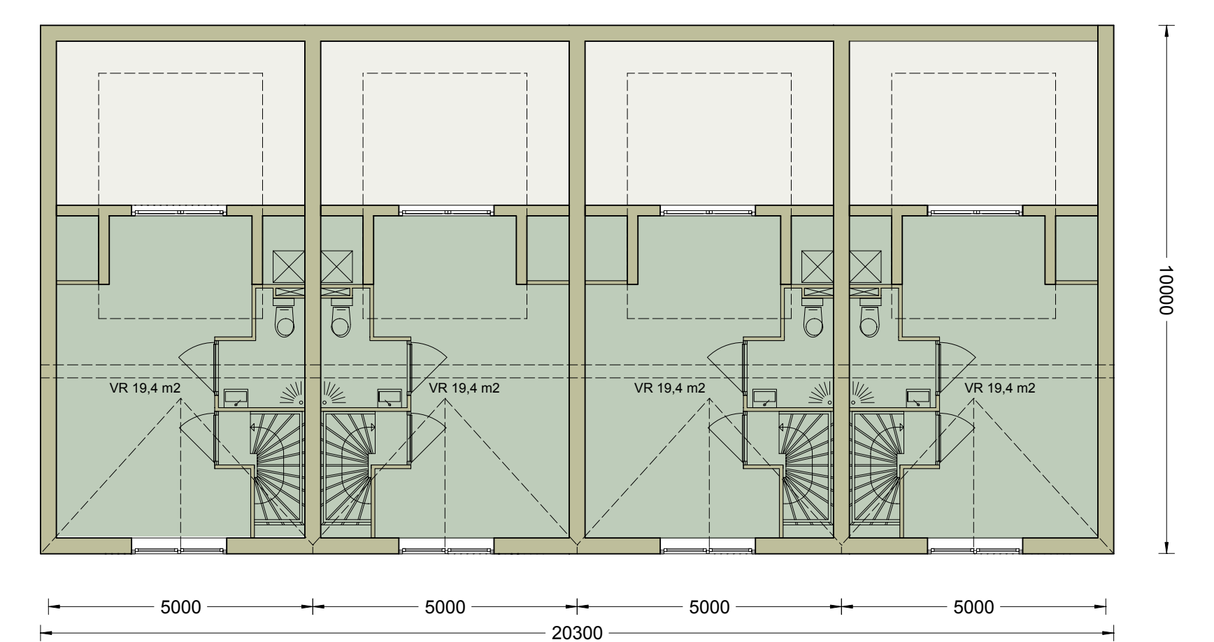
2e verdieping
