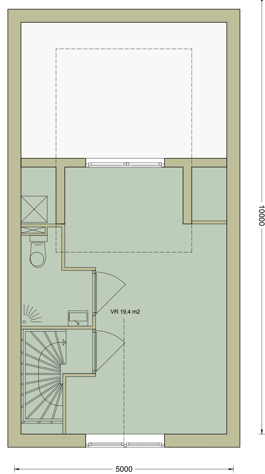
2e verdieping-Variant 2
