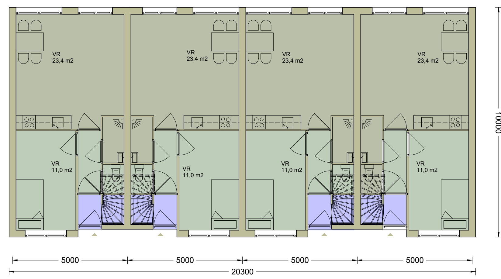
Begane grond
