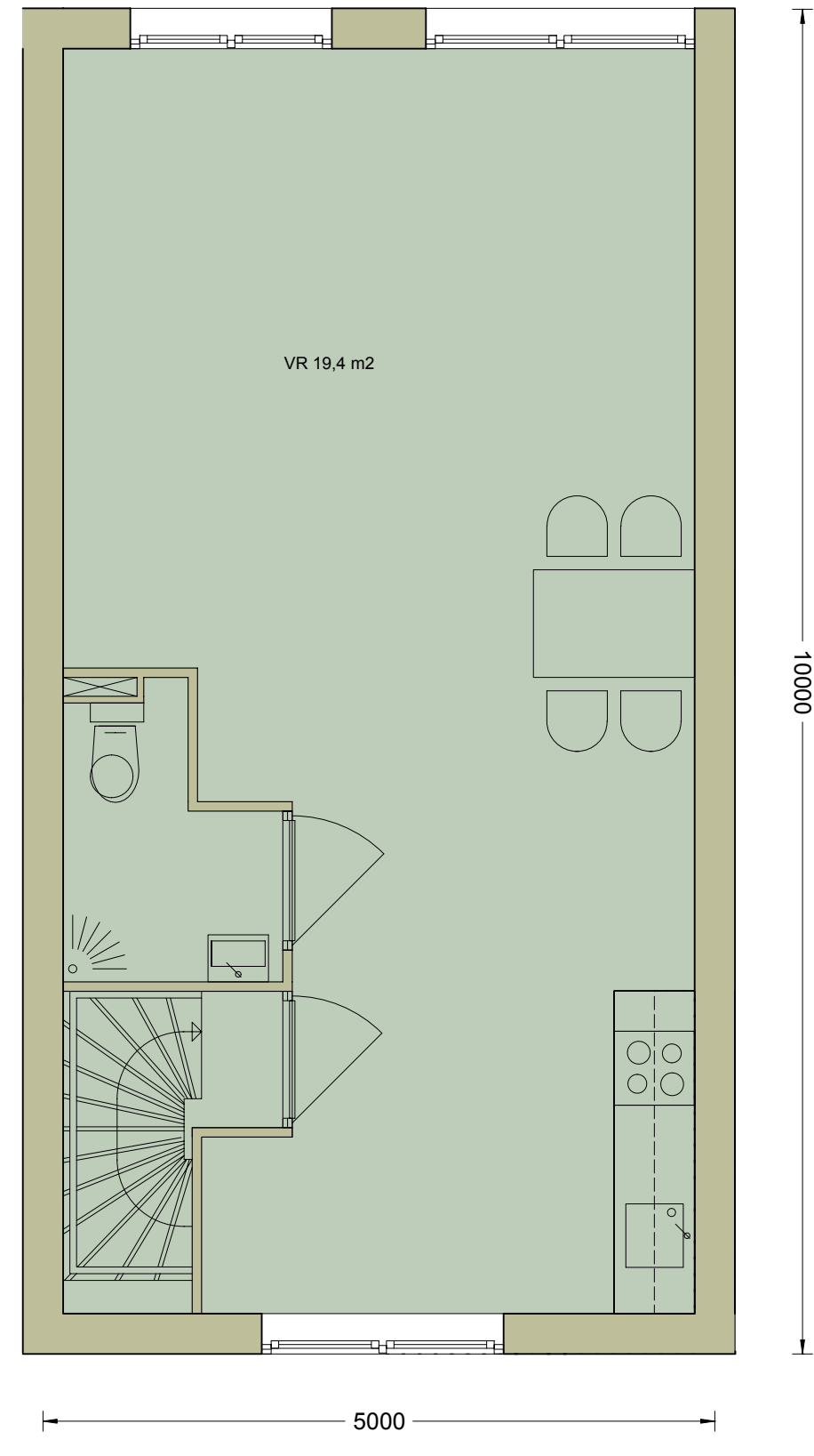
1e verdieping
