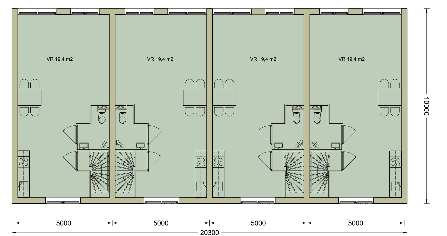
1e Verdieping
