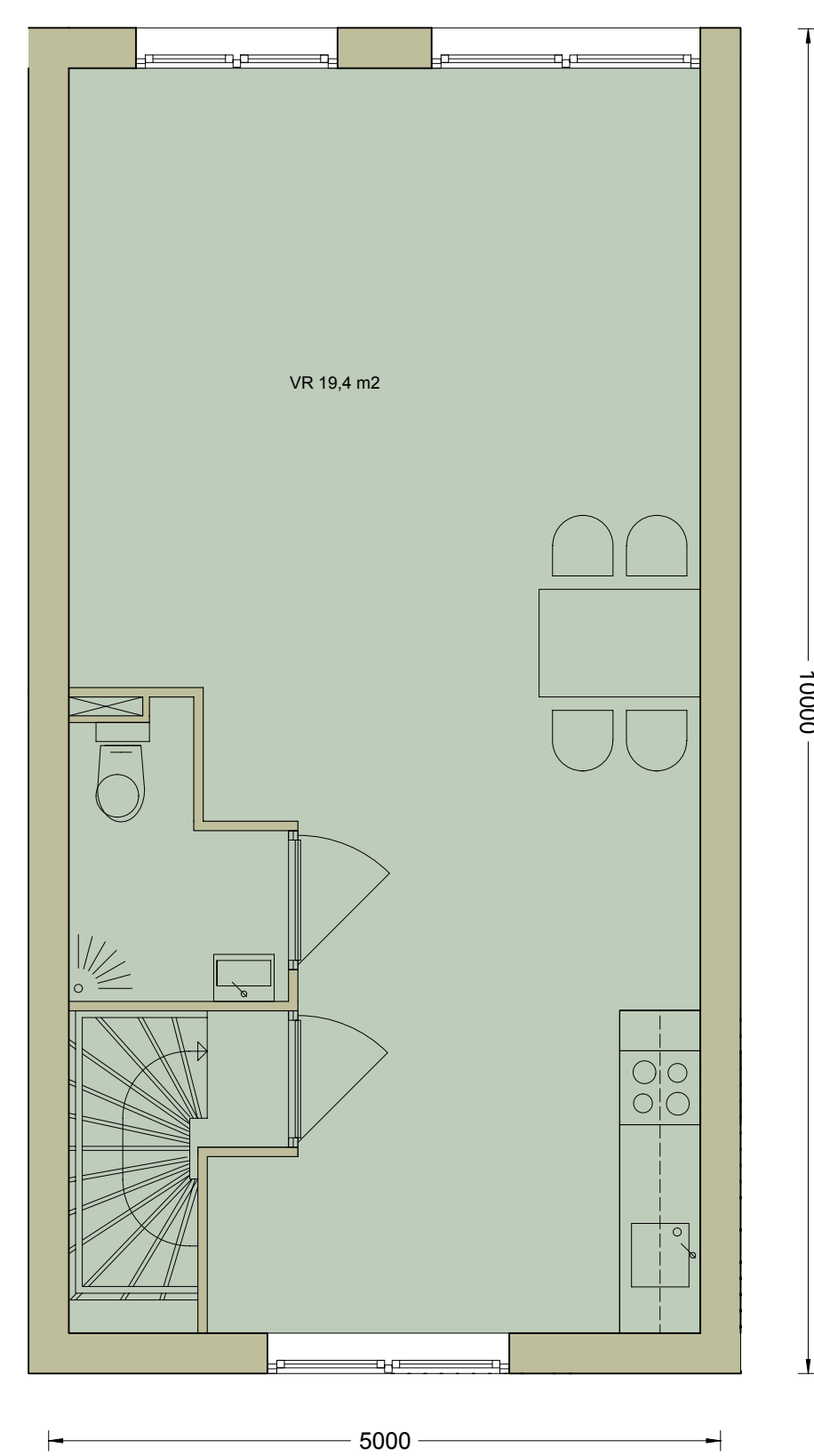
1e verdieping-Variant 2
