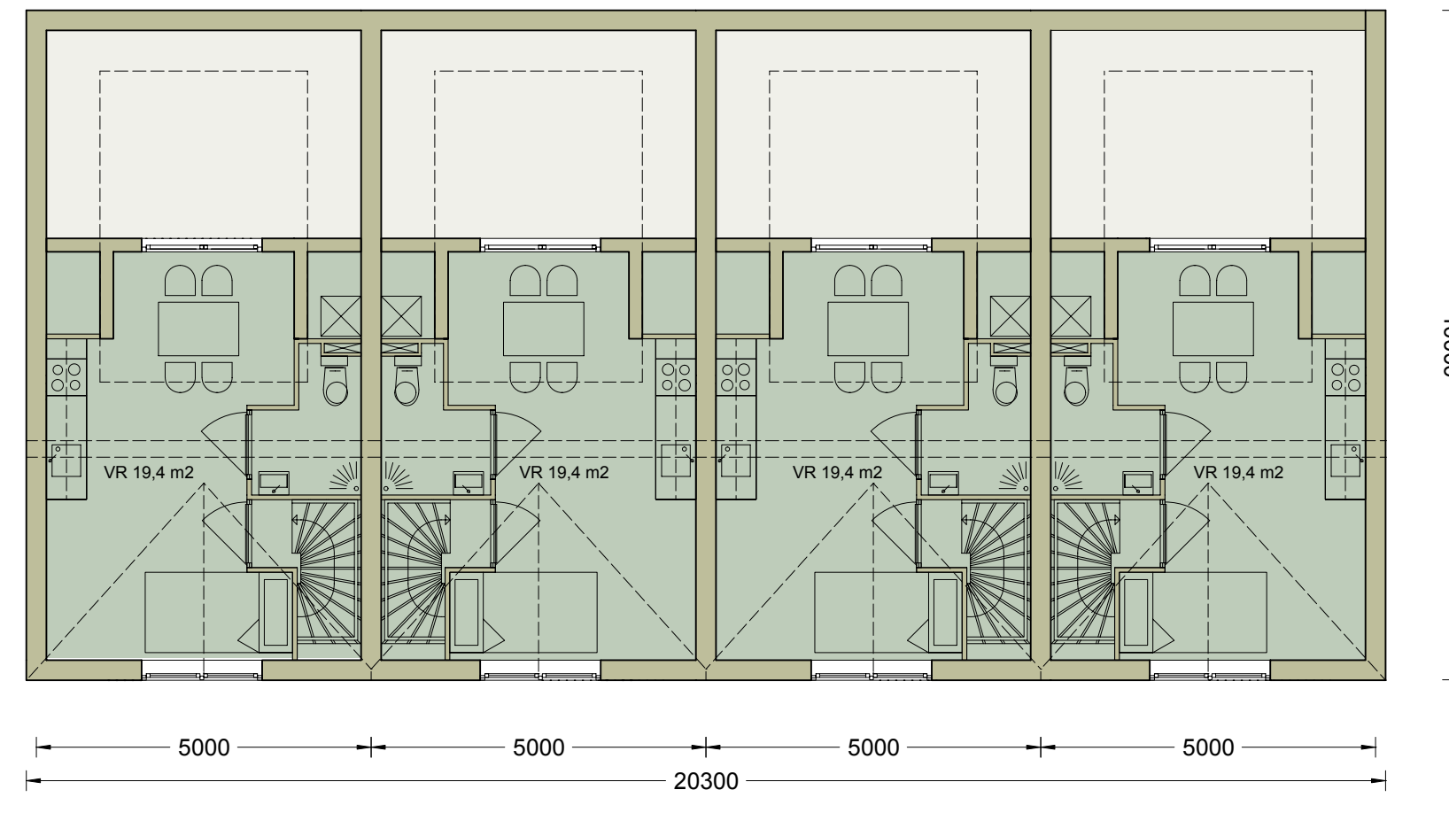
1e Verdieping
